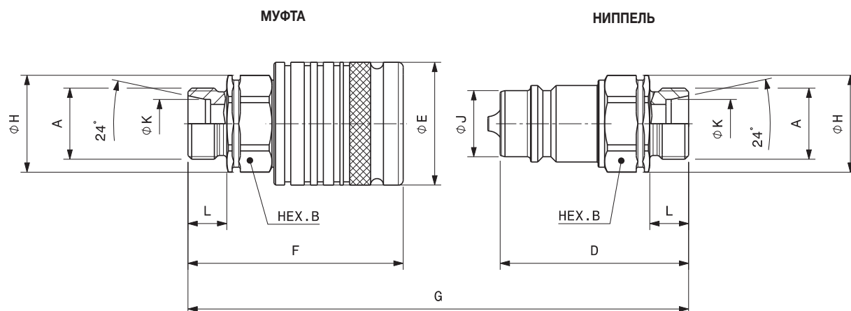
Описание порта: НАРУЖНАЯ РЕЗЬБА МЕТРИЧЕСКАЯ L СЕРИЯ -24 КОНУС (ISO 8434-1 и DIN 2353)
